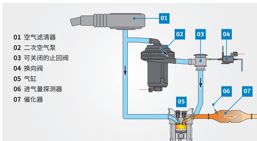
二次进气喷射系统原理（气动控制）
