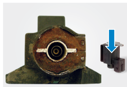
腐蚀的换向阀（已打开）
