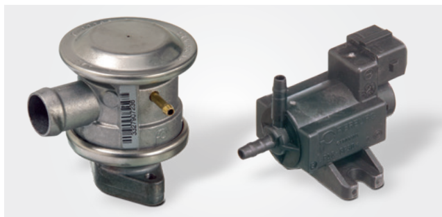
真空控制的关闭/止回阀 （从 1995 年左右）与换向阀
